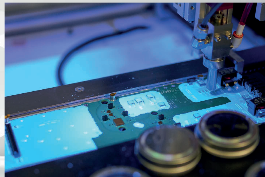
Робототехническая система нанесения влагозащитных материалов PVA Delta 6.
